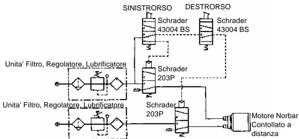
Circuito ad aria per l'azionamento destrorso o sinistrorso del motore controllato a distanza
