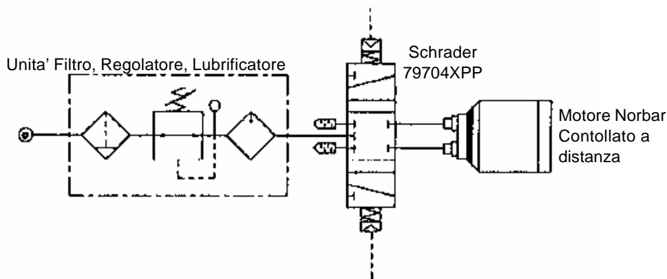
Circuito di controllo per l'azionamento del motore controllato a distanza tramite il segnale elettrico a distanza
